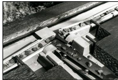
Bild 13: Plattenband im Modell
