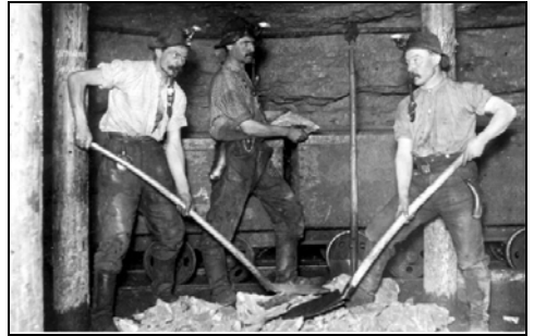
Füllen der Förderwagen in der Abbaustrecke
